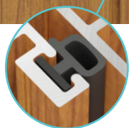
Vista Elegante Por Vinil VHP en Contramarco
