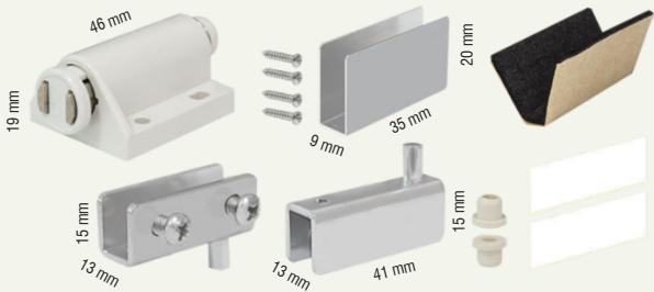
Bisagra, Contra Push y Contra Imán
