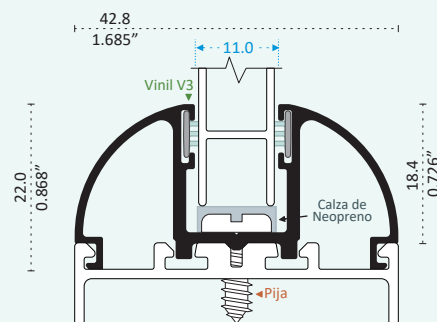
34323 PATENTE SOLISTA Longitud: 6.10 m
