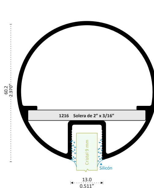
23896 PATENTE PASAMANOS 2.3" Longitud 6.10 m
