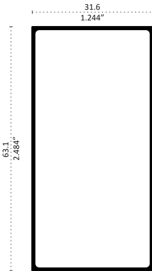
62513 RECTANGULAR 2 1/2" x 1 1/4" Longitud 6.10 m
