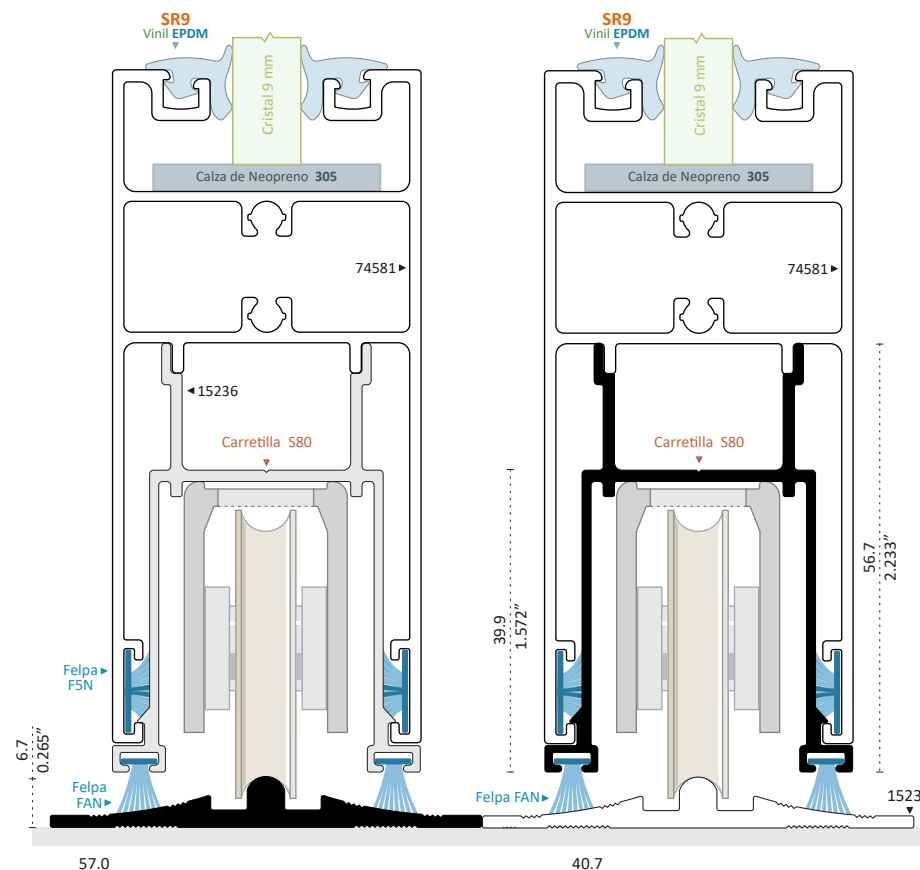
15231 PATENTE RIEL SENCILLO Longitud 6.10 m
