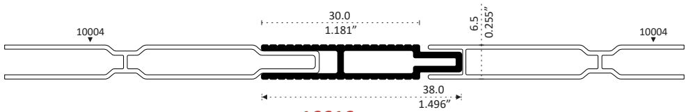
16616 DUELA ESTRIADA DOBLE VISTA Longitud : 6.10 m
