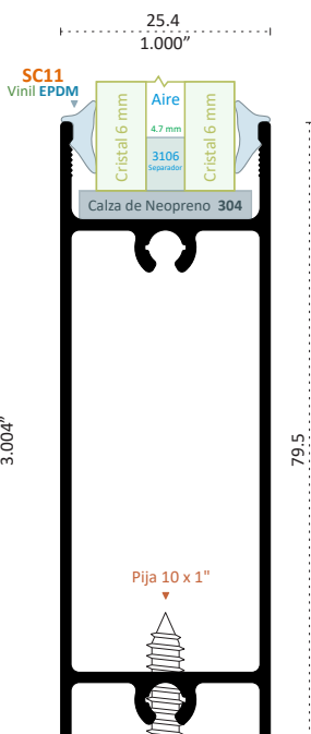
9962 ZOCLO CON BASE Longitud 6.10 m
