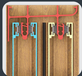
Riel Doble Opcional Dos Hojas Móviles
