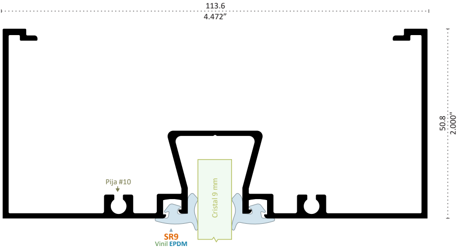
13614 BOLSA Longitud 6.10 m
