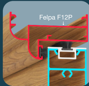
Mayor Hermeticidad y Aislamiento entre Batiente y Cabezal por sus Dos Felpas
