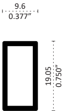
2502 RECTANGULAR 3/4" x 3/8" Longitud 6.10 m
