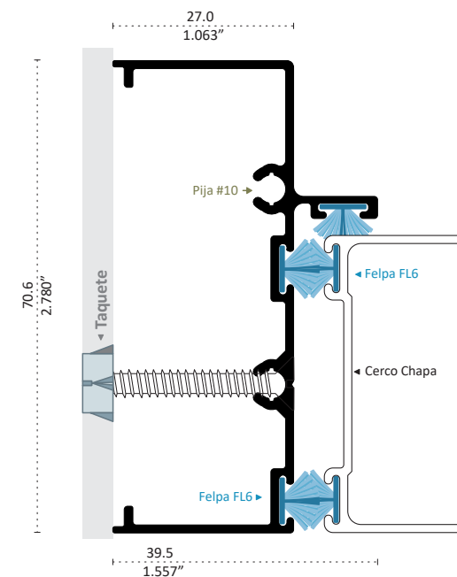
12757 BATIENTE Longitud 6.10 m
