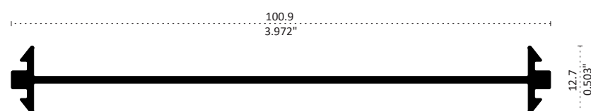
23577 MOLDURA UNIÓN Longitud 6.10 m
