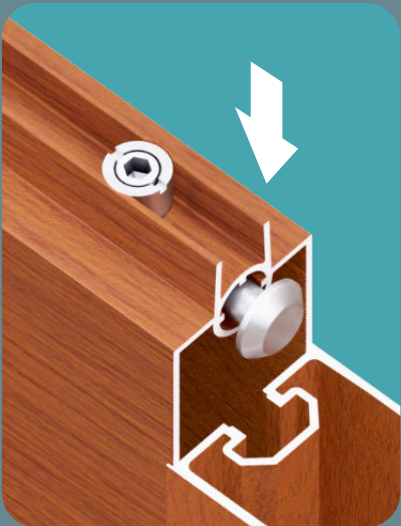
Opresores para Mayor Rapidez en el Armado
