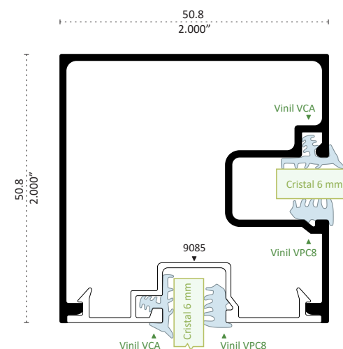
8586 ESQUINERO Longitud 6.10 m
