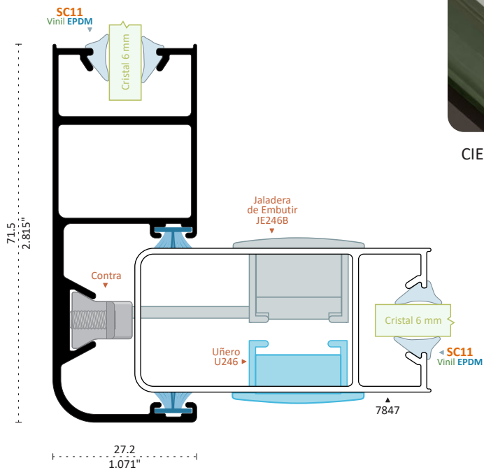
7849 ESQUINERO Longitud 6.10
