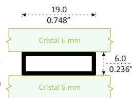
15043 CUADRÍCULA AMERICANA Longitud 6.10 m
