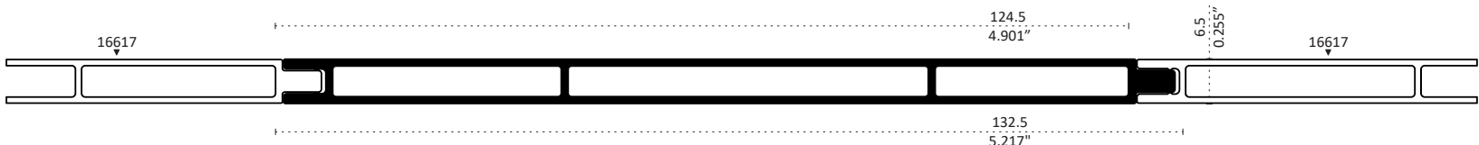
16617 PATENTE DUELA LISA DOBLE VISTA 5" Longitud : 6.10 m 16617-5 5.00 m 16617-C 4.60 m
