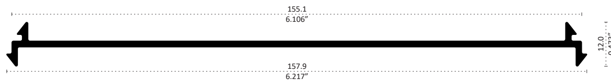
23618 MOLDURA UNIÓN Longitud: 6.10 m
