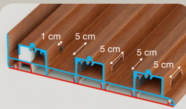
Riel Inferior Incluye Drenes cada 40 cm Colocar Felpa F11P
