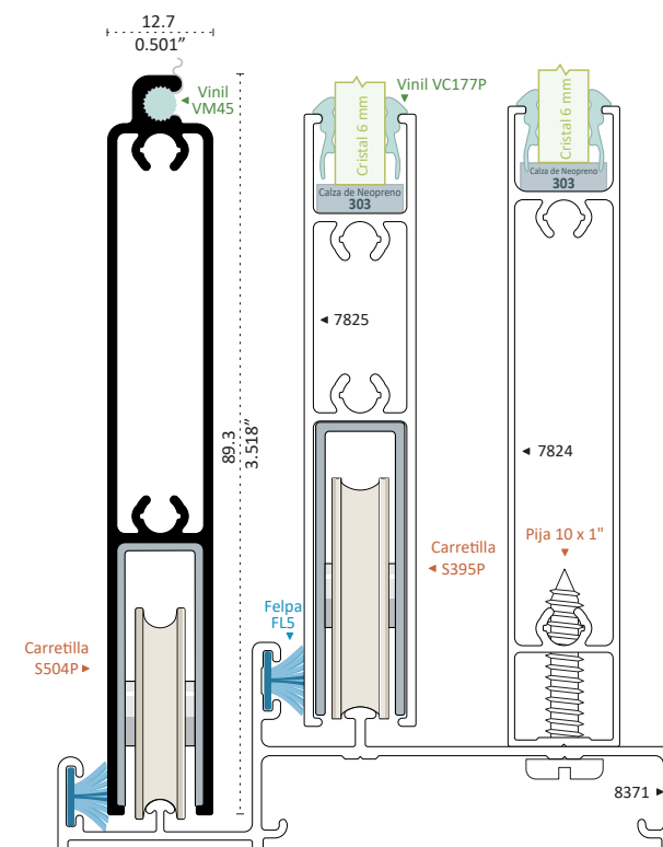
16533 PATENTE MOSQUITERO HORIZONTAL GRAN VISTA Longitud 6.10 m
