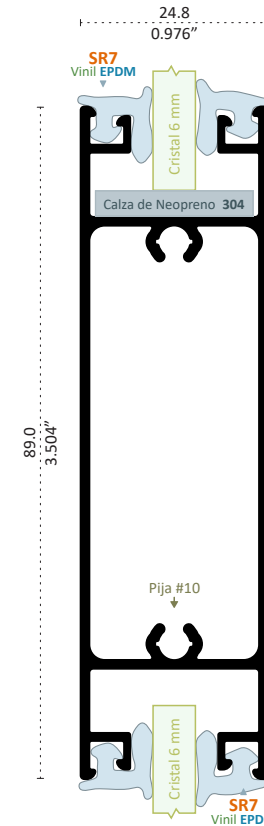
68411 INTERMEDIO Longitud 6.10 m
