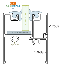
Línea Fija Serie 35
