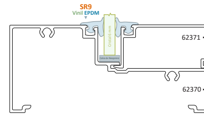
Línea Fija Serie 70 Triple
