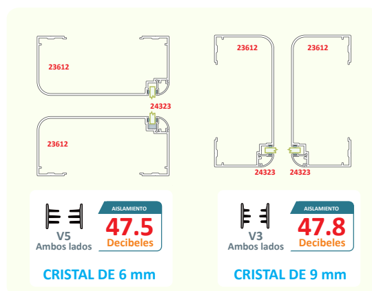
23612 ESCALONADO CURVO DESCENTRADO Longitud 6.10 m
