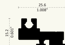
12538 BARRA DE ARMADO Longitud 3.03 m PARA PERFILES: MB33 9187 MB57 19187 MB107 412596
