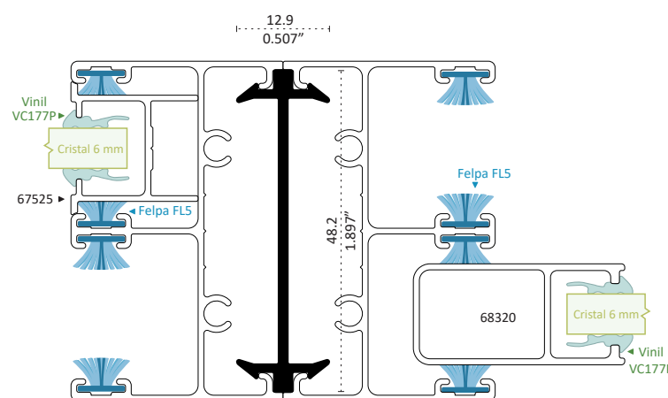
7792 MOLDURA UNIÓN Longitud 6.10 m
