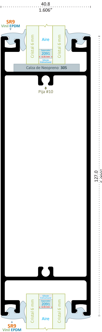
24410 INTERMEDIO 5" Longitud 6.10 m
