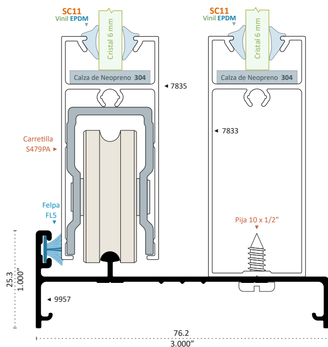
9957 RIEL Longitud 6.10 m
