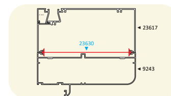
23630 MOLDURA UNIÓN Longitud 6.10 m
