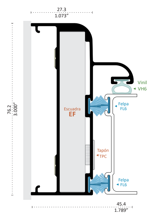
9110 BATIENTE Longitud 5.50 m
