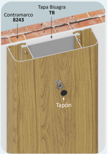
Fijación de Contramarco a Muro
