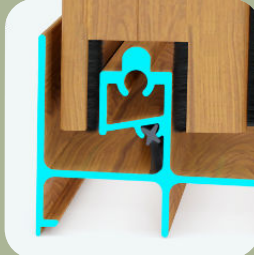
2 Felpas Verticales en Traslapes
