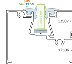
Línea Fija Serie 50
