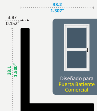
21311 Longitud 6.10 m
