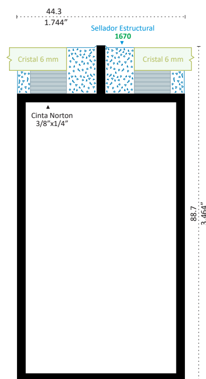
611003 BÁSICO TUBULAR INTEGRAL 3" X 1 3/4" Longitud 6.10 m
