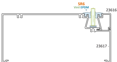
Línea Fija Serie 100 Triple Cristal de 6 mm
