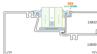
Línea Fija Serie 80 Cristal Doble Riel Triple
