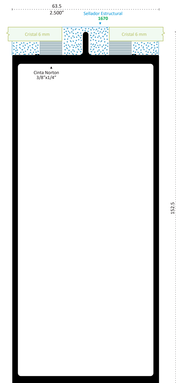
14739 BÁSICO TUBULAR INTEGRAL 6" X 2 1/2" Longitud 6.10 m
