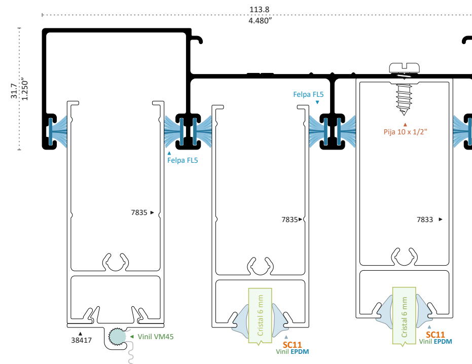
7863 CONTRAMARCO MOSQUITERO CORREDIZO SIN VENAS Longitud 6.10 m
