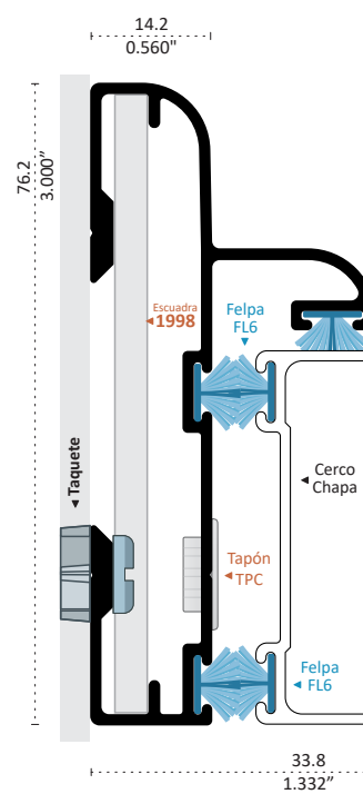
9244 BATIENTE COLONIAL Longitud 6.10 m
