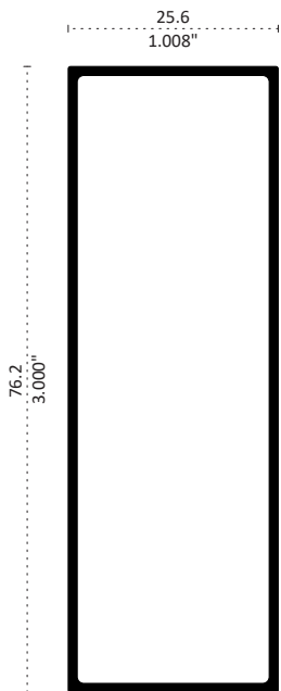
62516 RECTANGULAR 3" x 1" Longitud 6.10 m
