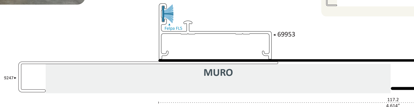
9247 PATENTE REPIZÓN CAPFCE Longitud 6.10 m 9247-C 4.00 m
