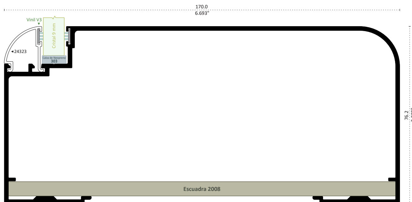
23612 ESCALONADO CURVO DESCENTRADO Longitud 6.10 m
