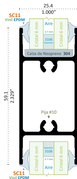
9961 INTERMEDIO Longitud 6.10 m
