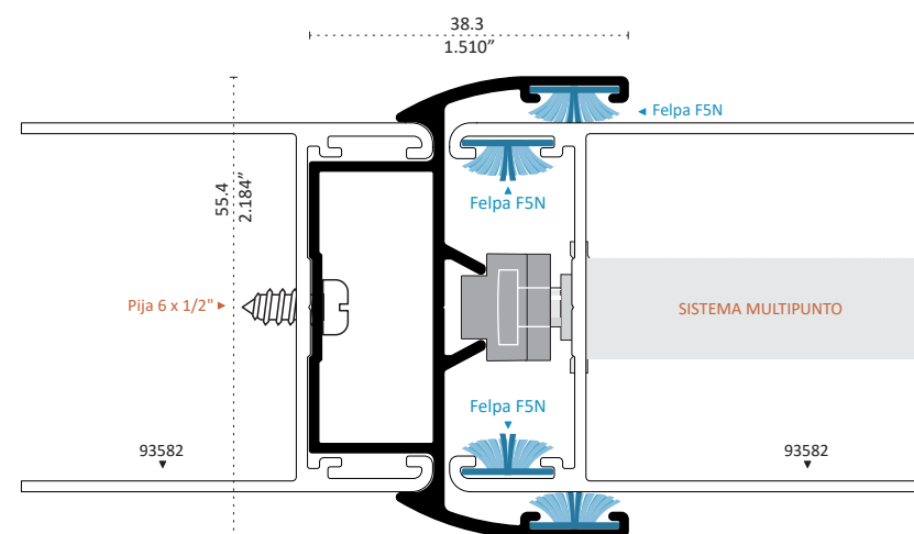
33637 ADAPTADOR Longitud 6.10 m
