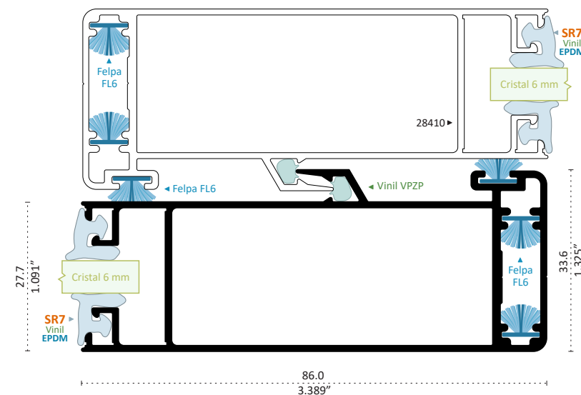
28410 PATENTE TRASLAPE PUERTA Longitud 5.00 m 28410-L 6.10 m
