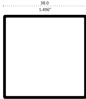
2363 CUADRADO 1 1/2" Longitud 6.10 m
