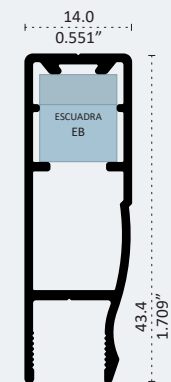
9756 PATENTE MARCO Longitud 6.10 m
