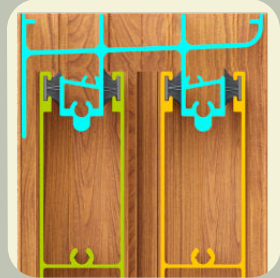
Riel Doble Opcional Dos Hojas Móviles
