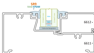
Línea Fija Serie 70 Cristal Doble
