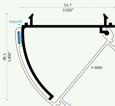
9089 PATENTE ESQUINERO REGULABLE Longitud 6.10 m 9089-C 3.05 m
