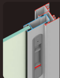
Cerco 11048 Recibe Broche de Embutir 914
