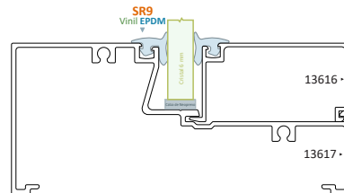
Línea Fija Serie 80 Triple Cristal de 9 mm
