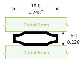
12393 CUADRÍCULA INGLESA Longitud 6.10 m
