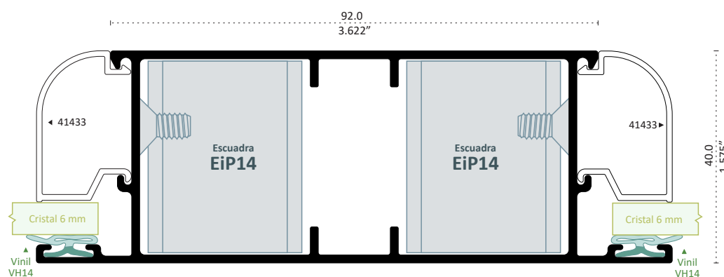
41423 PILASTRA GRAN VISTA Longitud 6.10 m
