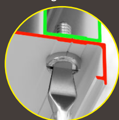
Pijas sin Contacto con el Cristal
