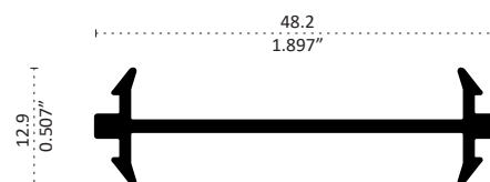
7792 MOLDURA UNIÓN Longitud 6.10 m
