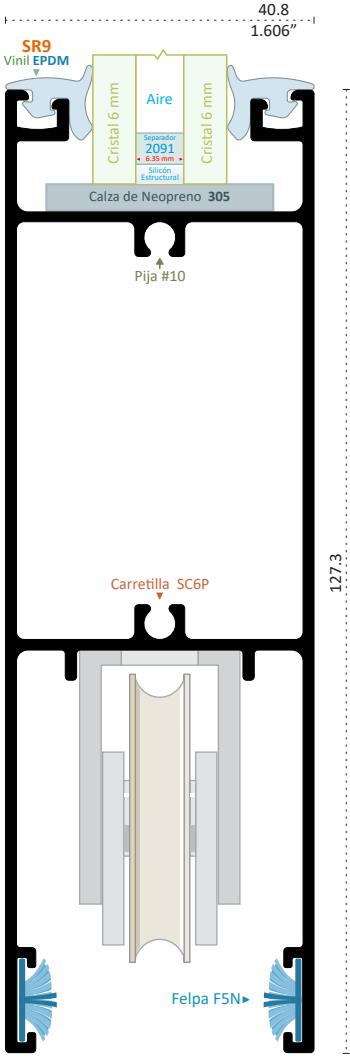
34082 ZOCLO CABEZAL Longitud 6.10 m
