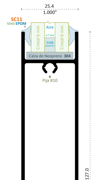
19959 ZOCLO Longitud 6.10 m
