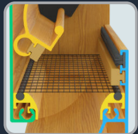
Mosquitero Horizontal Oculto
