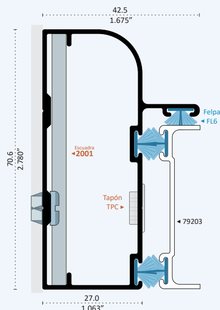
22757 PATENTE BATIENTE COLONIAL Longitud 6.10 m
