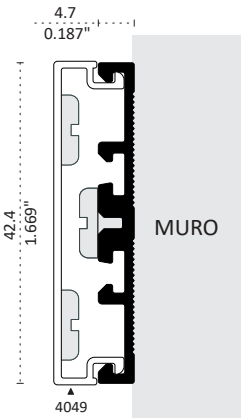
14322 PORTA JUNQUILLOS Longitud 6.10 m
