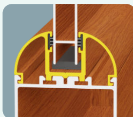
34323 PATENTE SOLISTA Longitud: 6.10 m
