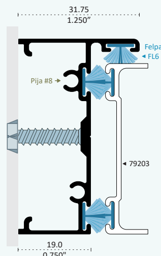
55844 BATIENTE Longitud 6.10 m
