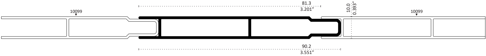
10099 PATENTE DUELA PARKET DOBLE VISTA Longitud : 6.10 m 10099-C 3.05 m 10099-5 5.00 m
