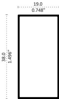
62515 RECTANGULAR 1 1/2" x 3/4" Longitud 6.10 m
