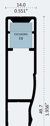
6854 MARCO Longitud 6.10 m
