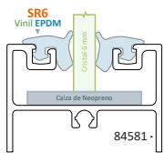
Serie 100 Cristal de 6mm
