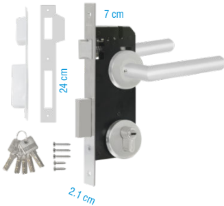
2822 Llave - Llave
