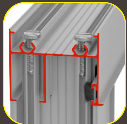
Contramarco de Dimensiones Correctas
