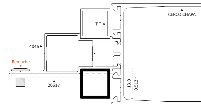
2361 CUADRADO 13 mm Longitud 6.10 m
