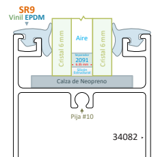
Serie 100 Cristal Doble
