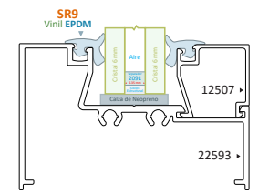
Línea Fija Serie 70 y 80 Cristal Doble
