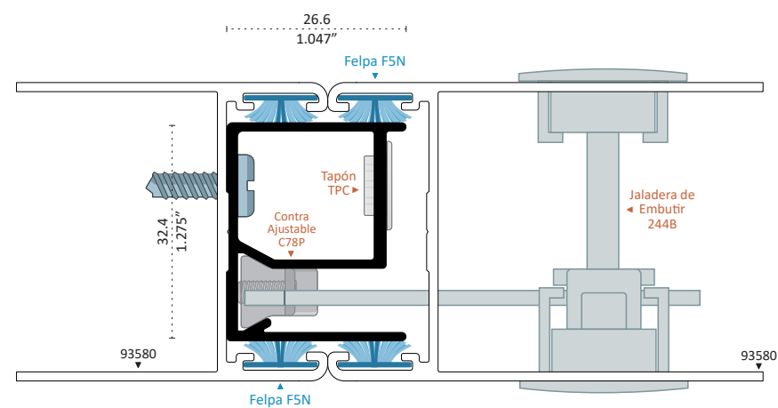
13637 PATENTE ADAPTADOR Longitud 6.10 m
