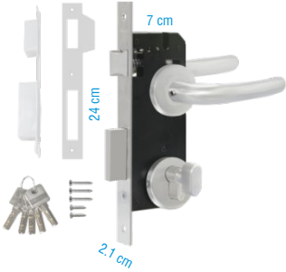
2867 Llave - Mariposa
