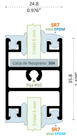
13842 PATENTE INTERMEDIO Longitud 6.10 m
