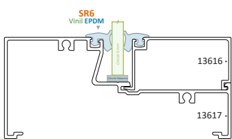
Línea Fija Serie 100 Cristal de 6 mm
