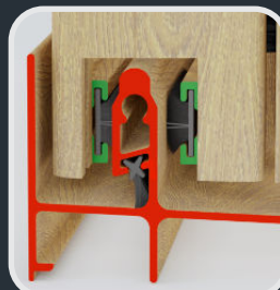
2 Felpas Horizontales en Zoclo
