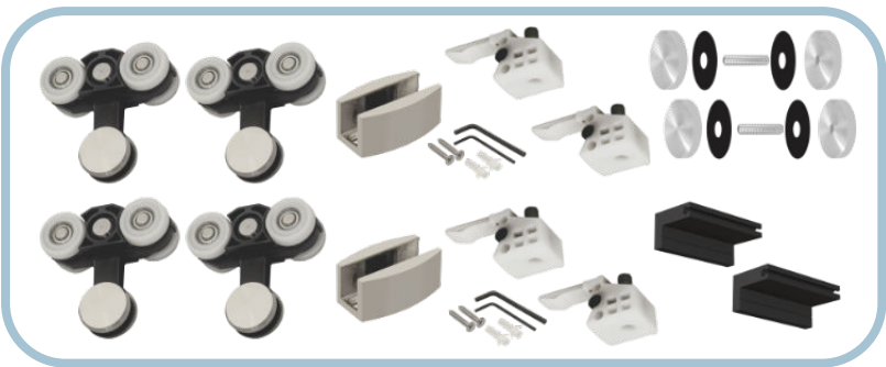
SE REQUIEREN 2 JUEGOS POR CANCEL JCT6 Juego para Cristal de 6 mm JCT9 Juego para Cristal de 9 mm
