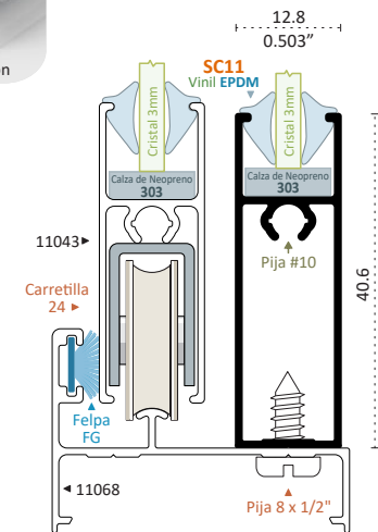
511046 PATENTE ZOCLO CON BASE Longitud 6.10 m
