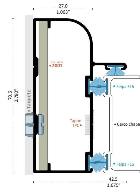
22757 PATENTE BATIENTE COLONIAL Longitud 6.10 m
