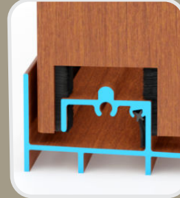
2 Felpas Verticales en Traslapes
