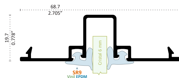
32505 TAPA BOLSA Longitud 6.10 m
