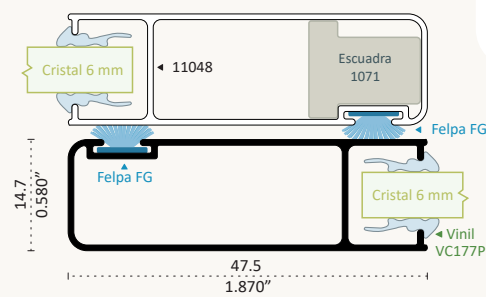
Traslape Altura Máxima 2.10 m
