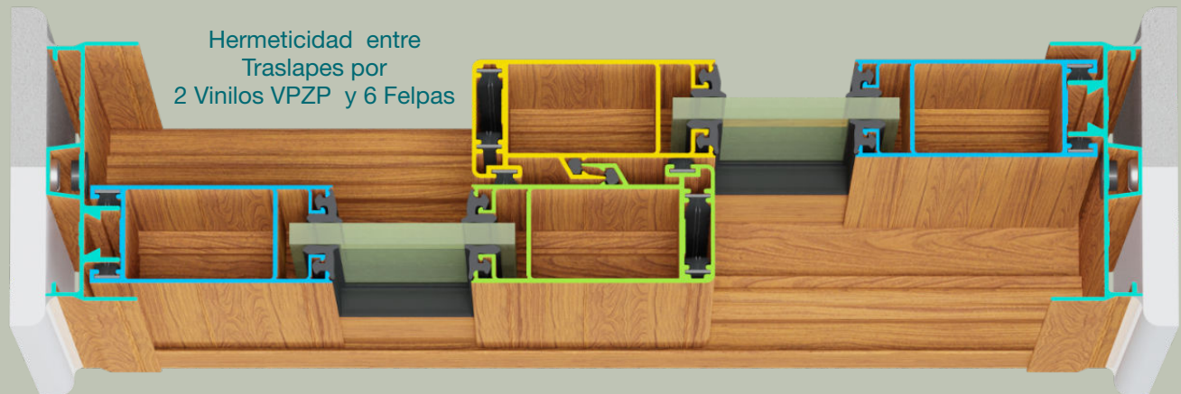
2 Felpas Horizontales en Zoclo
