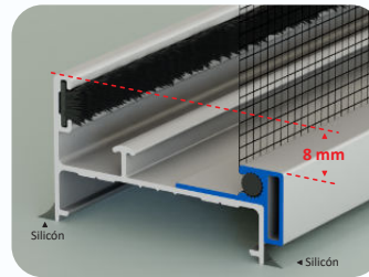
Mosquitero 7336 en Riel
