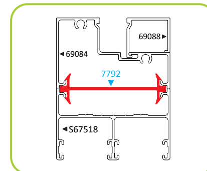
7792 MOLDURA UNIÓN Longitud 6.10 m
