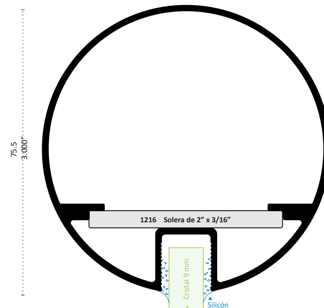
11559 PATENTE PASAMANOS 3" Longitud 6.10 m 11559-C 4.60 m
