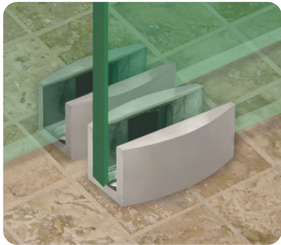
GUIA INFERIOR
