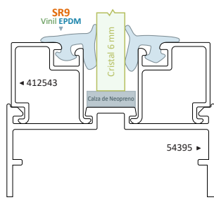
Junquillos Puerta Multidiseños
