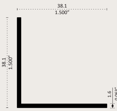
1420 Longitud 6.10 m
