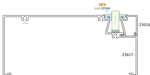
Línea Fija Serie 100 Triple
