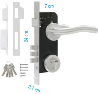
2865 Mecanismo de 3 Pasadores Llave - Llave
