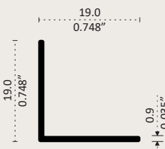
1303 Longitud 6.10 m
