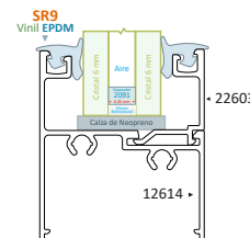
Línea Fija Serie 35 Cristal Doble
