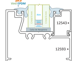
Línea Fija Serie 50 Cristal Doble
