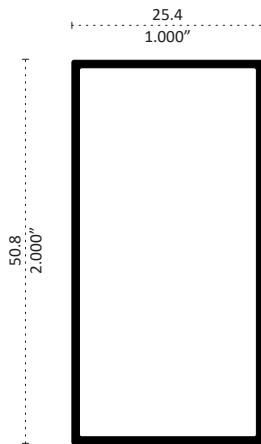
62521 RECTANGULAR 2" x 1" Longitud 6.10 m
