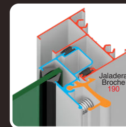
Cerco 11047 y Jaladera Broche 190
