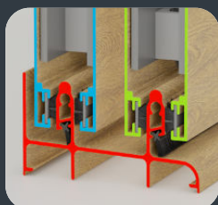
Riel con 4 Puntos de Apoyo
