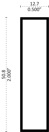
62508 RECTANGULAR 2" x 1/2" Longitud 6.10 m
