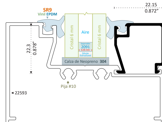
12507 JUNQUILLO Longitud 6.10 m
