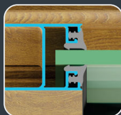
Vinilos Respaldo Mayor Firmeza por su Diseño Vinil Por Ambos Lados Aumenta Aislamiento Acústico
