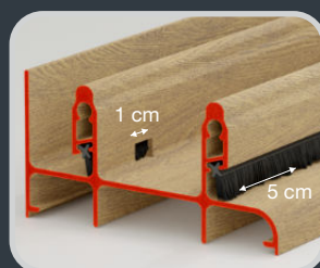
Riel Inferior Incluye Drenes cada 40 cm Colocar Felpa F11P
