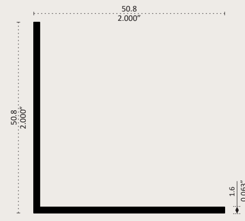
1421 Longitud 6.10 m
