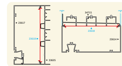
23618 MOLDURA UNIÓN Longitud: 6.10 m
