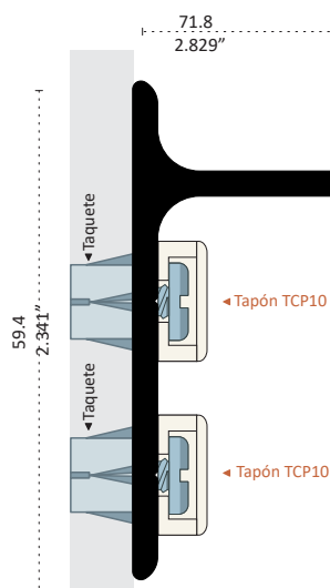
11560 PATENTE SOPORTE PASAMANOS Longitud 6.10 m
