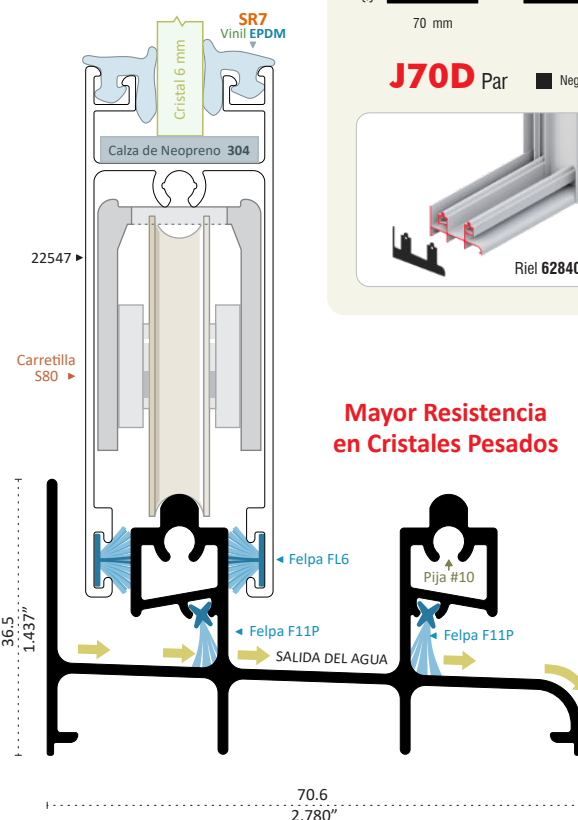
628407 PATENTE RIEL Y CABEZAL Longitud 6.10 m 628407-C 3.05 m
