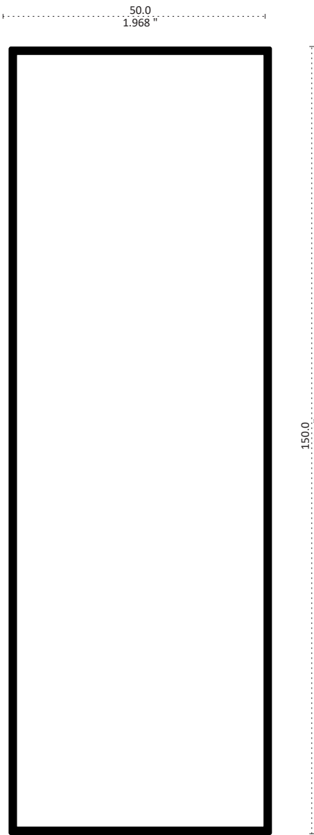
2533 VIGA Longitud 6.10 m Espesor 1.3 mm
