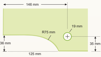
Resaque Pivote Inferior
