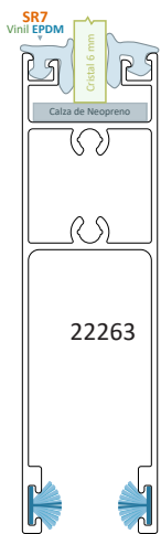
Corrediza Serie 70
