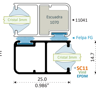
Traslape Altura Máxima 1.20 m
