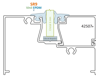
Línea Fija Serie 70 y 80
