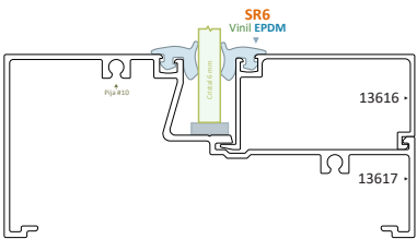
Línea Fija Serie 80 Triple
