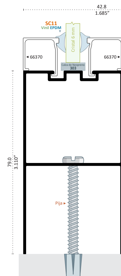
9131 ZOCLO FIJO LIGHT Longitud 6.10 m
