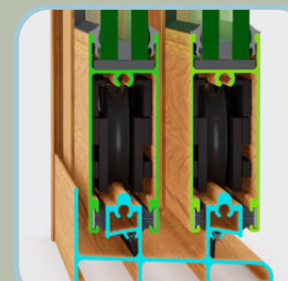
Doble Cristal de 6 mm con Separador de 3/16" Vinil en Ambos Lados
