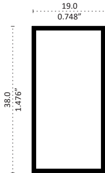
2515 RECTANGULAR 1 1/2" x 3/4" Longitud 6.10 m
