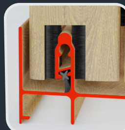
2 Felpas Verticales en Traslapes
