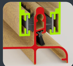
Mayor Hermeticidad por Doble Felpa entre Zoclo y Riel
