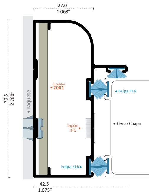
22757 PATENTE BATIENTE COLONIAL Longitud 6.10 m
