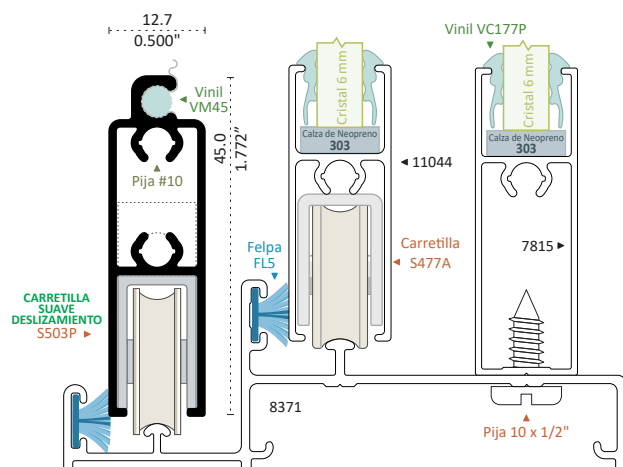
6533 PATENTE MOSQUITERO HORIZONTAL DOBLE VENA Longitud 6.10 m
