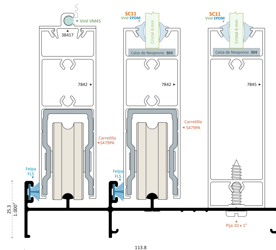
9275 RIEL MOSQUITERO INTERIOR Longitud 6.10 m
