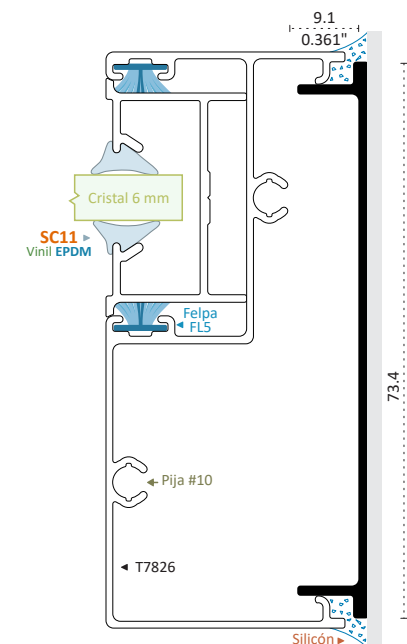
67317 MOLDURA DE FIJACIÓN Longitud 6.10 m TF3 10 cm
