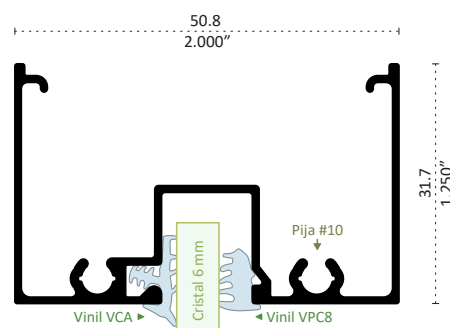
9083 PATENTE BOLSA Longitud 6.10 m
