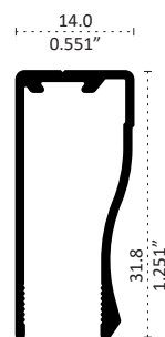
68802 MARCO Longitud 6.10 m 68802-C 3.66 m
