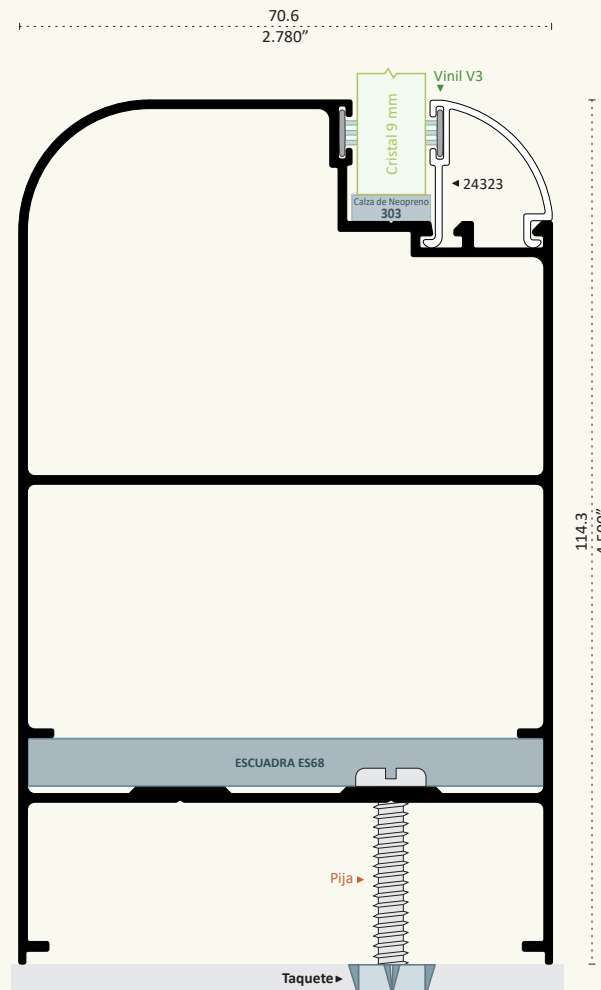
32508 PATENTE ESCALONADO GRAN VISTA Longitud 6.10 m (Armado a 45°)
