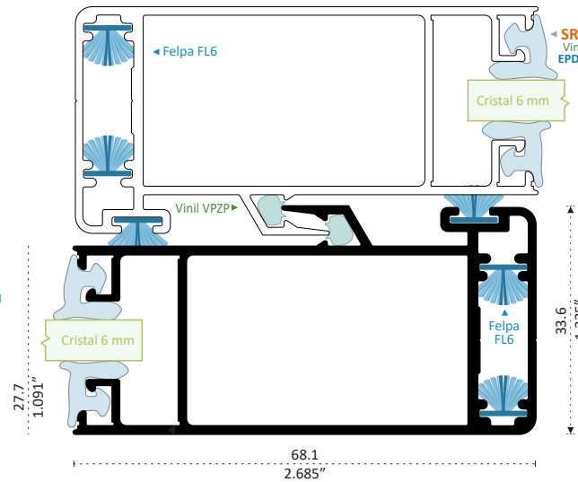
28412 PATENTE TRASLAPE VENTANA Longitud 6.10 m
