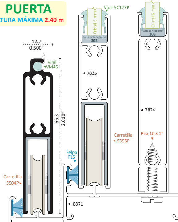
26533 PATENTE MOSQUITERO HORIZONTAL Longitud 6.10 m
