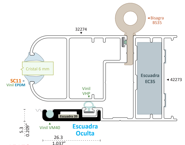
15173 MOSQUITERO FIJO Longitud 6.10 m
