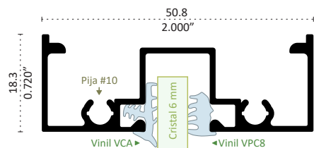
29086 BOLSA CORTA 2" TEMPLE T1 Longitud 6.10 m
