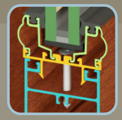
Adaptador Recibe 16 Junquillos
