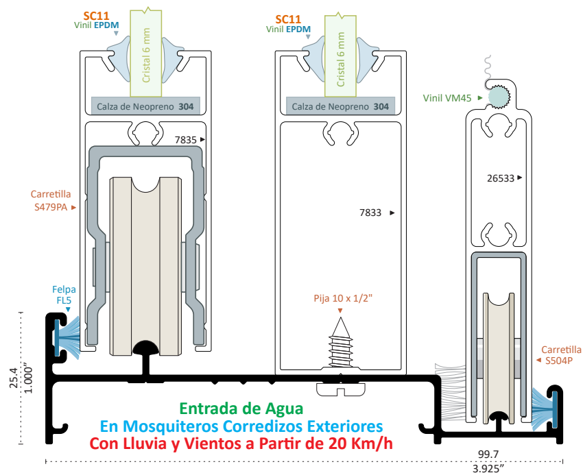
9272 PATENTE RIEL MOSQUITERO EXTERIOR Longitud 6.10 m
