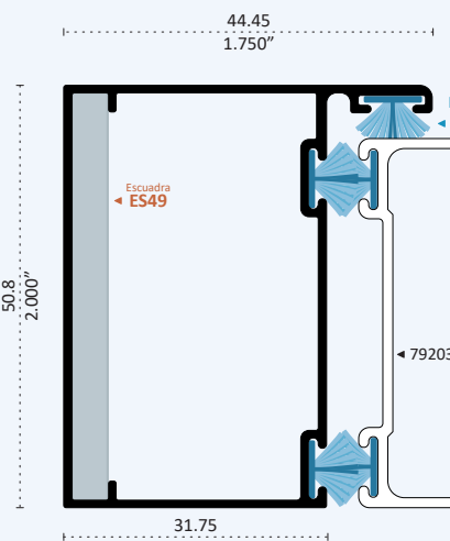
28591 PATENTE BATIENTE Longitud 6.10 m
