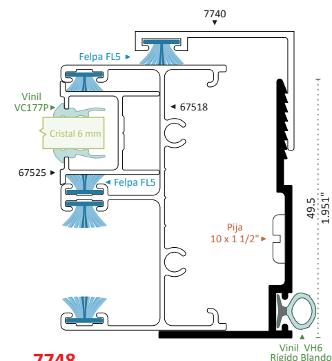
7748 BÁSICO AJUSTE VERTICAL Longitud 6.10 m
