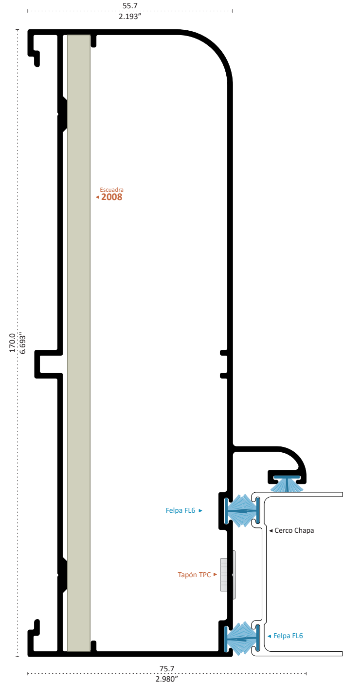
9243 BATIENTE COLONIAL Longitud 6.10 m
