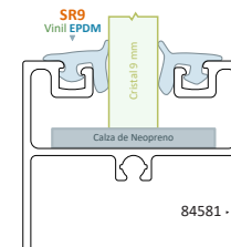
Serie 100 Cristal de 9 mm
