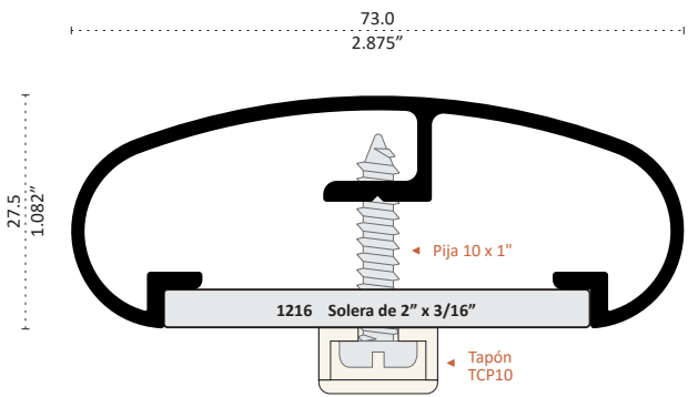
9366 PASAMANOS Longitud 6.10 m
