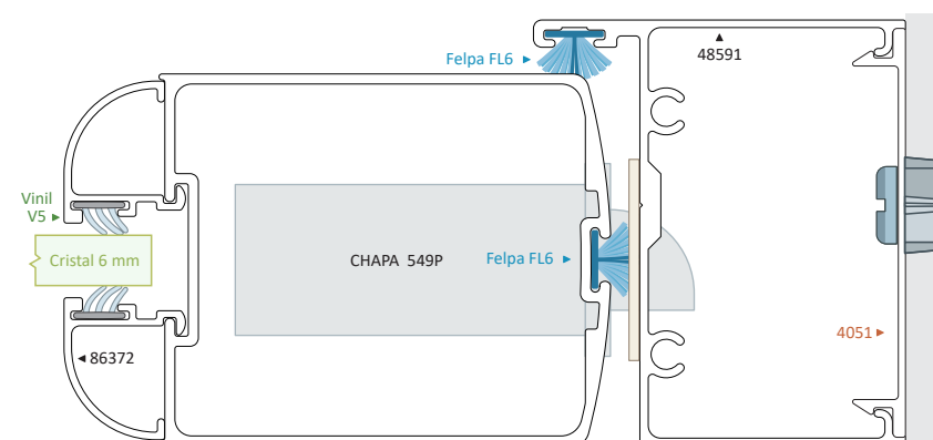
BSL32 Para Perfil 79187, 79183
