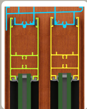
Riel Doble Opcional Dos Hojas Móviles
