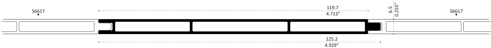
S6617 DUELA LISA DOBLE VISTA Longitud : 5.80 m
