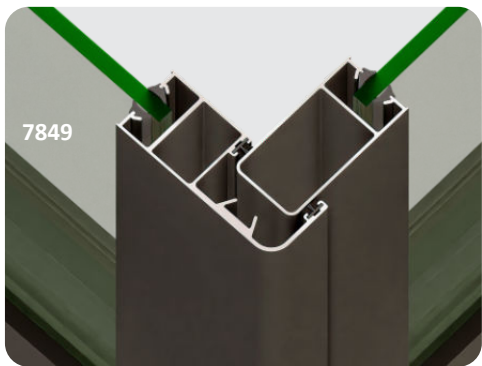
CIERRE DE ESQUINERO CON CERCO CHAPA
