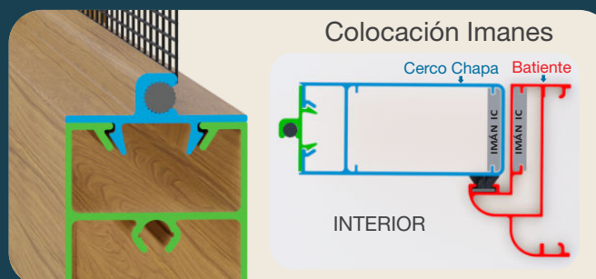
Adaptador Mosquitero
