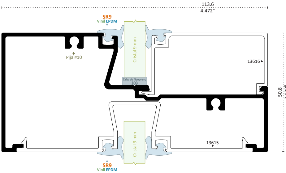
13617 ESCALONADO Longitud 6.10 m
