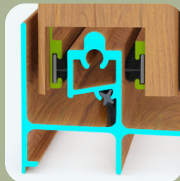
2 Felpas Horizontales en Zoclo
