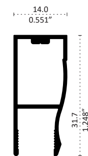
11036 MARCO Longitud 3.77 m
