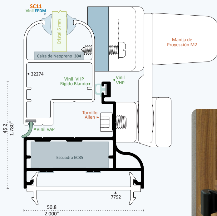
69091 PATENTE CONTRAMARCO Longitud 6.10 m
