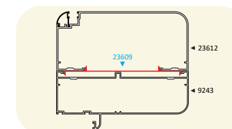
23609 MOLDURA UNIÓN Longitud 6.10 m
