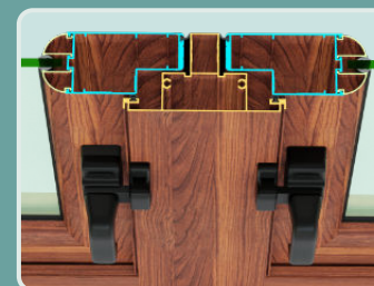
Intermedio Hojas Dobles
