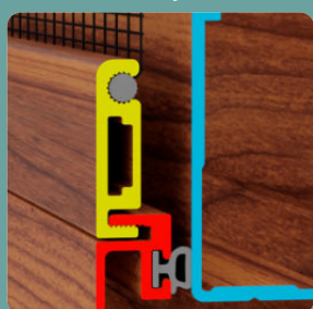
Con Estrías, Escuadra Oculta y Vinil Estriado para Mayor Agarre
