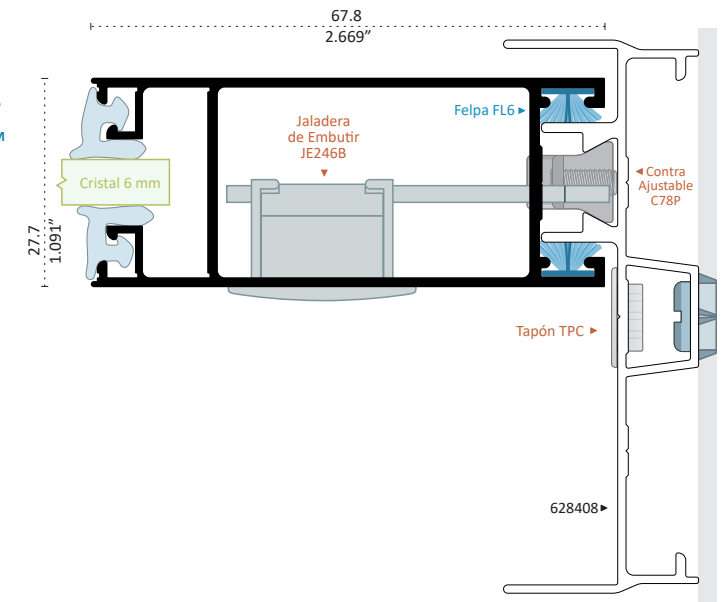
28411 PATENTE CERCO CHAPA VENTANA Longitud 6.10 m
