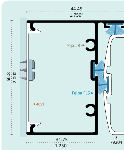
78591 PATENTE BATIENTE Longitud 6.10 m
