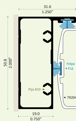
45844 BATIENTE Longitud 6.10 m
