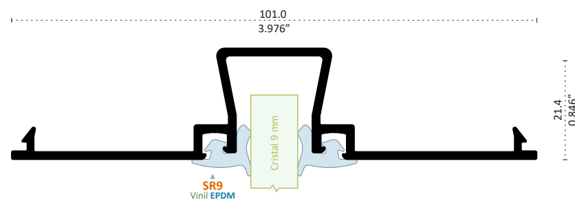
13615 TAPA BOLSA Longitud 6.10 m
