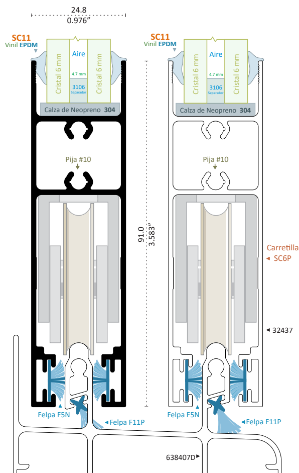
32437 PATENTE ZOCLO Y CABEZAL Longitud 6.10 m
