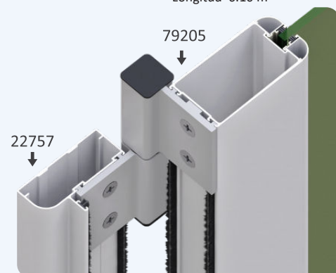
28591 PATENTE BATIENTE Longitud 6.10 m
