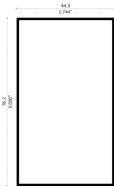
62522 RECTANGULAR 3" x 1 3/4" Longitud 6.10 m
